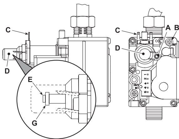
Рис. 15. Газовый клапан
