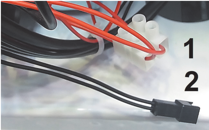
Рис. 7. Доступ к соединительным колодкам подключения комнатного термостата (1) и датчика температуры бойлера (2)
