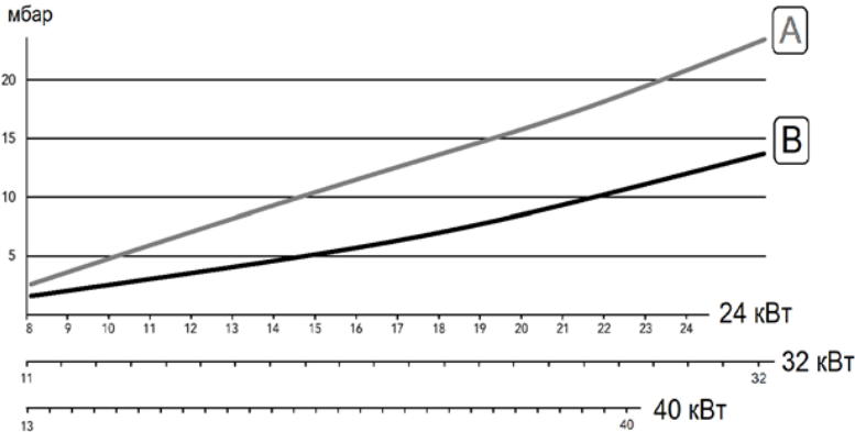
Давление газа/мощность
