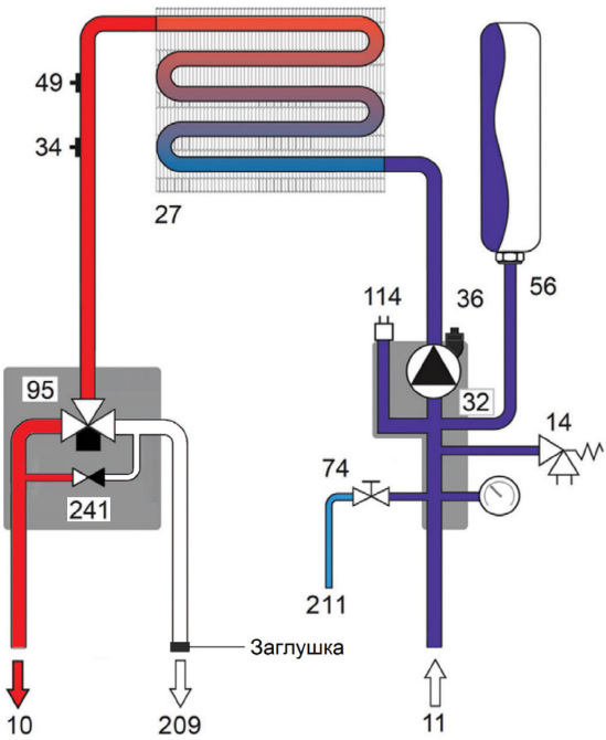
Рис. 18. Отопительный контур
