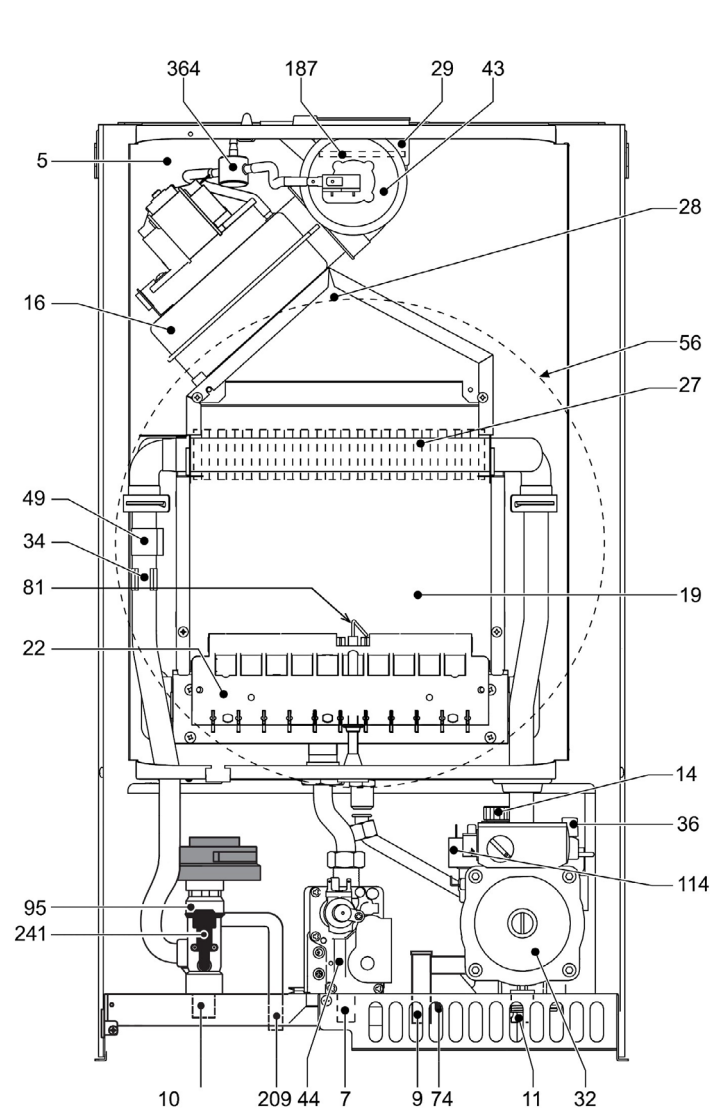
Рис. 176. Конструкция VITABEL HF 32/40
