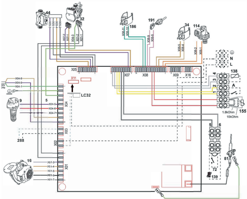
Рис. 45. Электрическая схема
