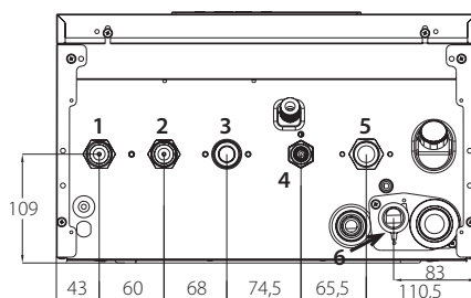
Рис. 35. Вид снизу
