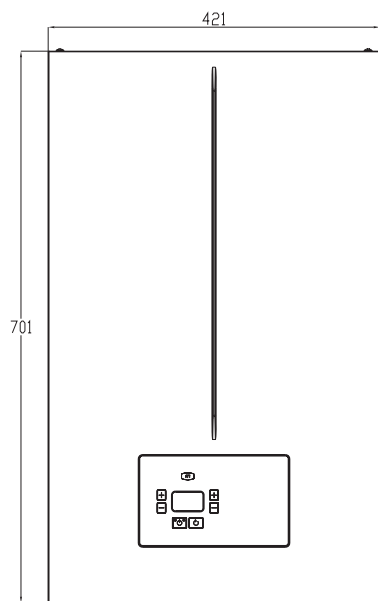
Рис. 36. Вид спереди
