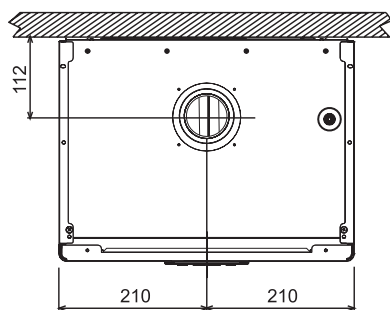
Рис. 38. Вид сверху
