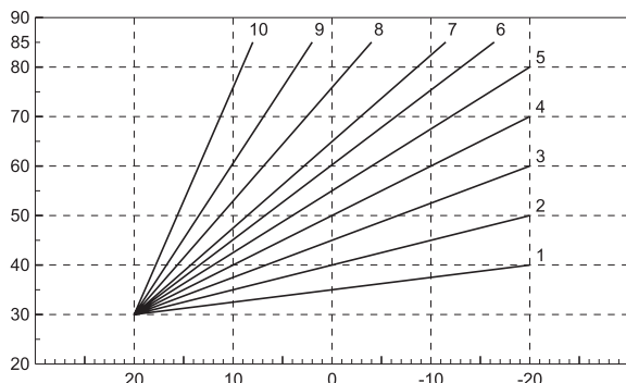
Рис. 14. Компенсационные кривые
