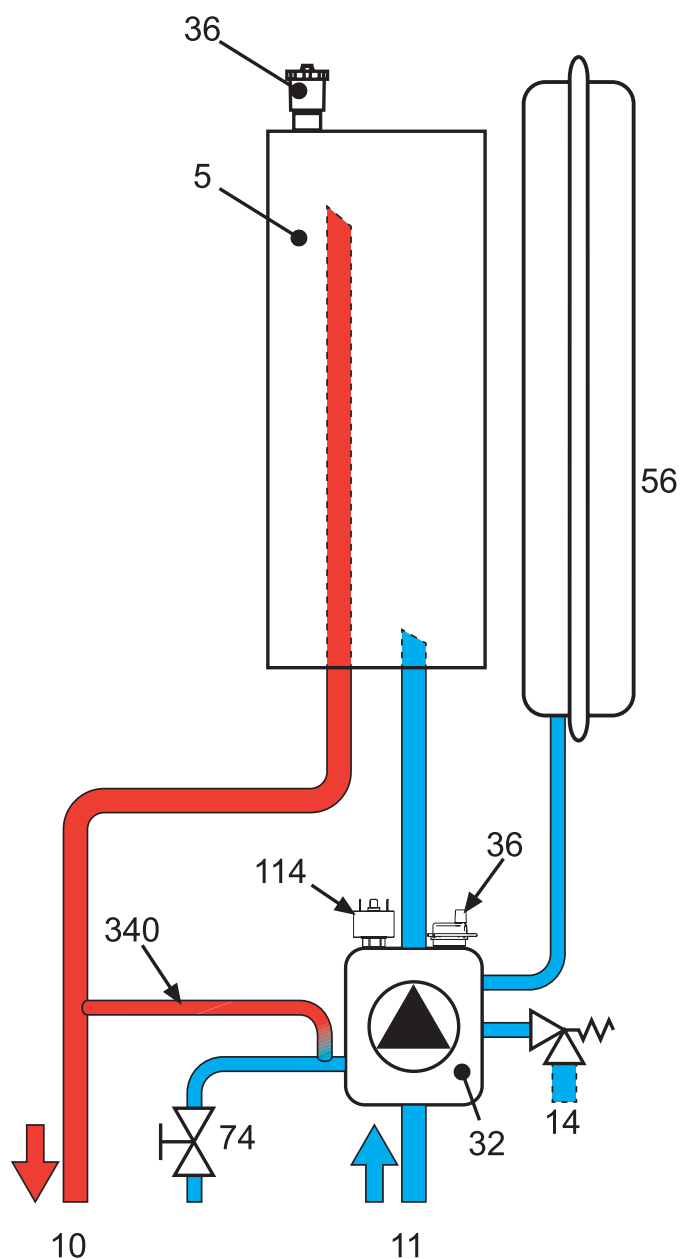
Рис. 16 Гидравлическая схема
