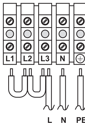
Рис. 20. Однофазная проводка
