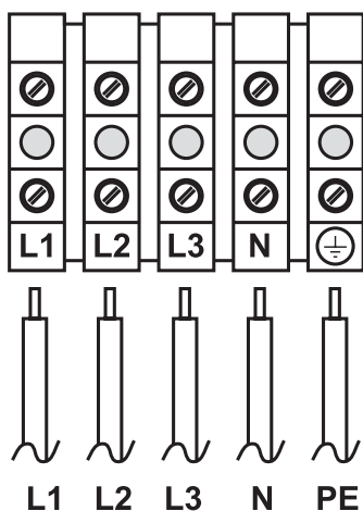
Рис. 19. Трехфазная проводка
