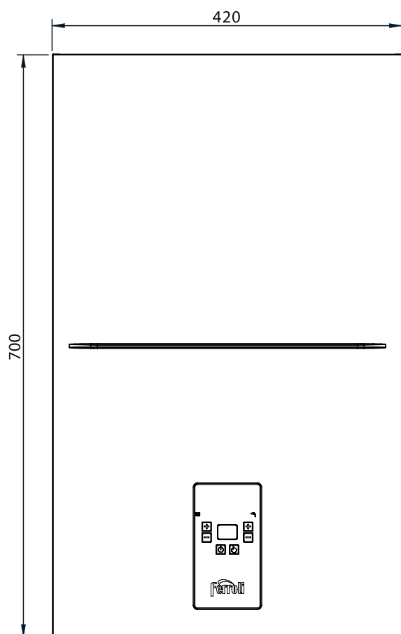
Рис. 10. Вид спереди
