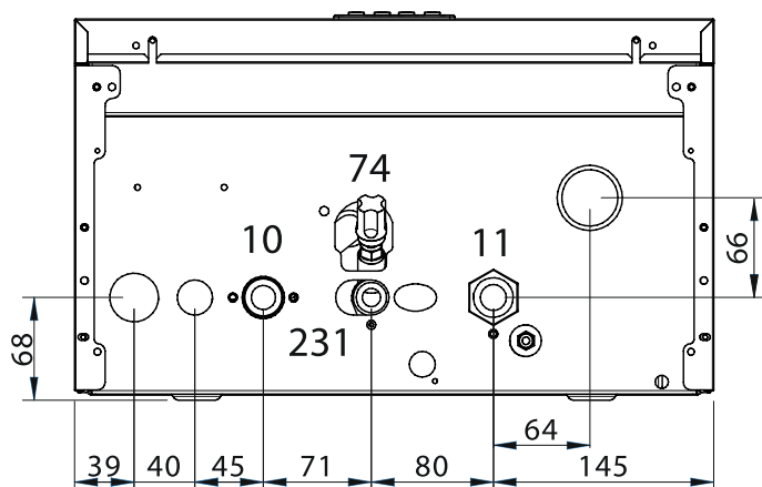
Рис. 12. Вид снизу
