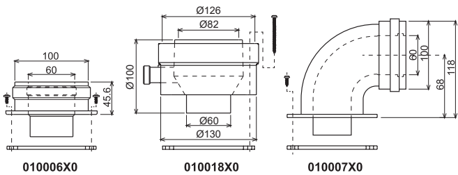
Рис. 9. Начальные элементы для коаксиальных воздуховодов
