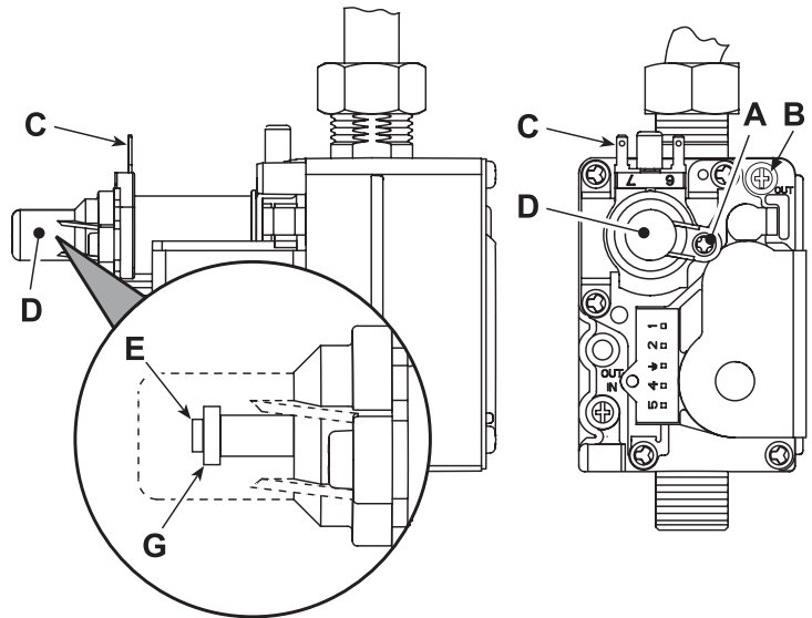
Рис. 15. Газовый клапан
