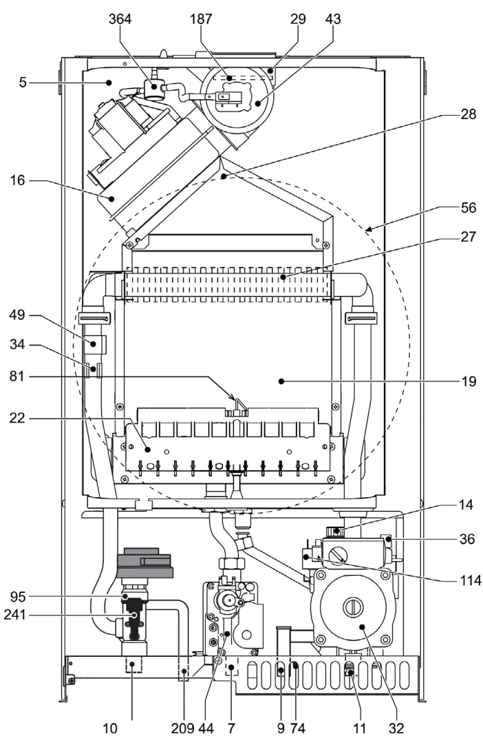
Рис. 17б. Конструкция VITABEL HF 32/40
