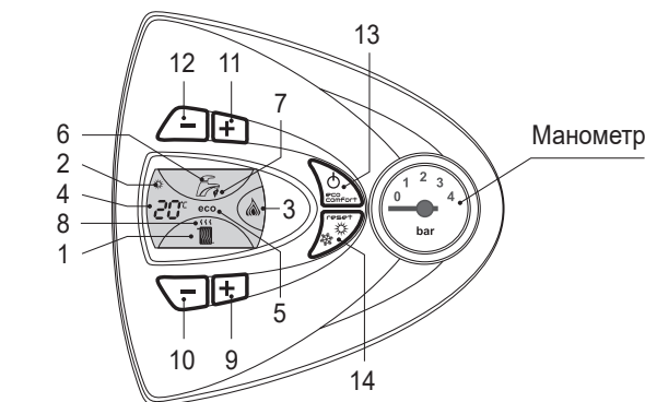
Рис. 1. Панель управления
