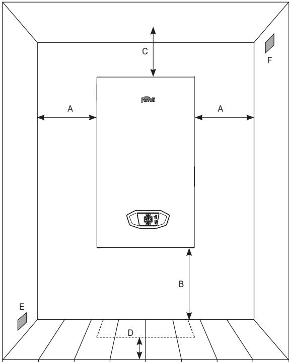
Рис. 3. Место установки
