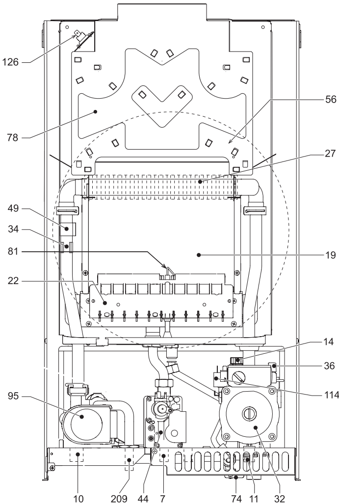
Рис. 17а. Конструкция VITABEL C
