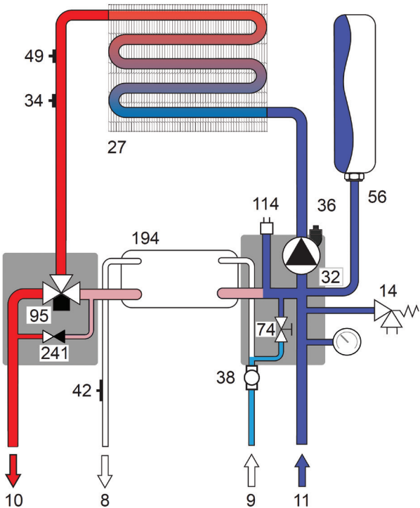
Рис. 18. Отопительный контур
