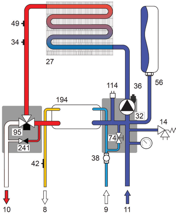
Рис. 19. Контур ГВС
