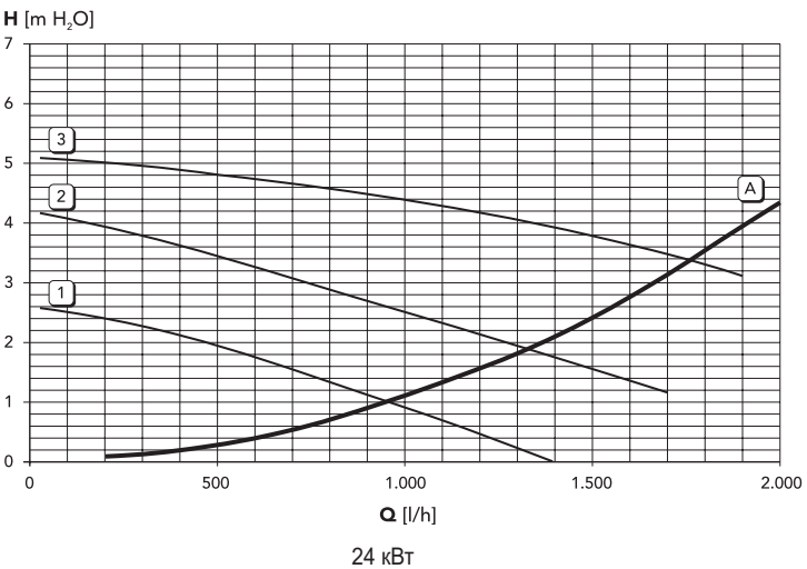
Потери напора циркуляционных насосов
