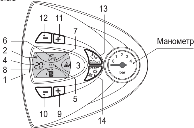
Рис. 1. Панель управления
