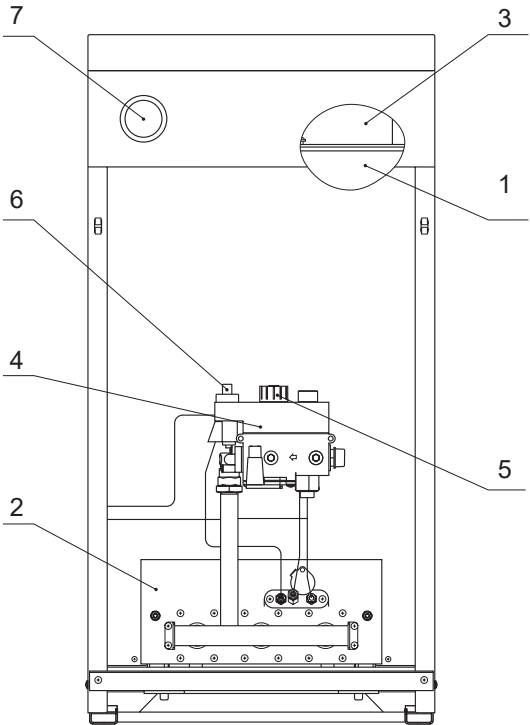
Рис. 3. Особенности котла с газовым блоком FERROLI 710 Модели котлов TORINO CLASSIC 25; 30
