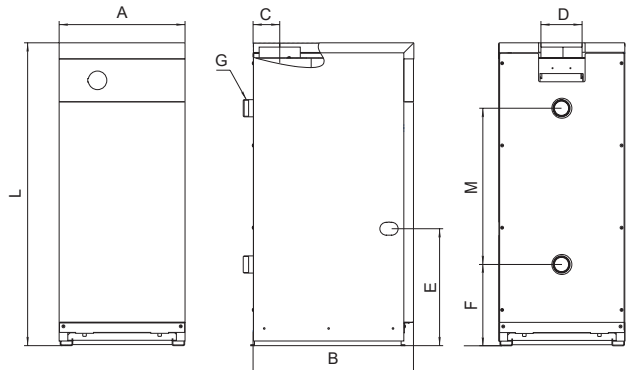
Рис. 1. Общий вид, габаритные и присоединительные размеры котлов
