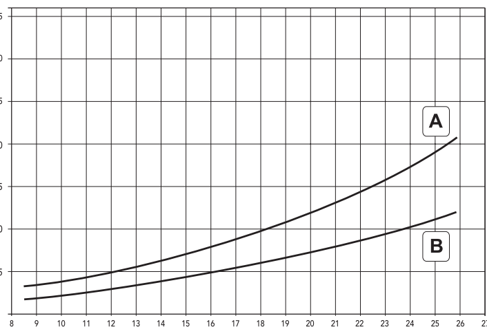
Рис. 16. Кривая давление газа/мощность А – сжиженный газ; В – метан
