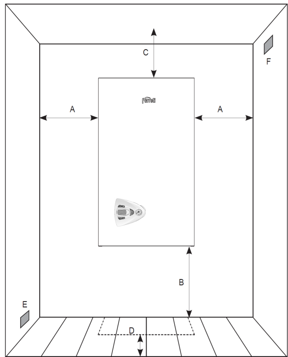
Рис. 3. Место установки
