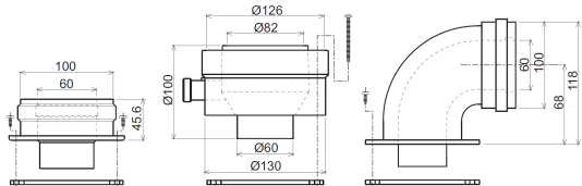
Рис. 8а. "Стартовые" элементы коаксиального дымохода
