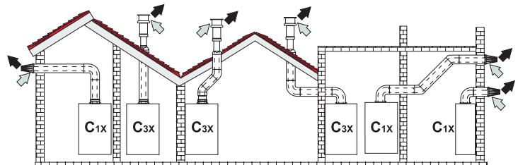
Рис. 7. Пример установки коаксиального дымохода (воздух/дым)
