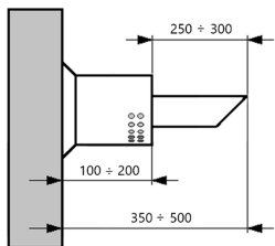
Рис. 8а. "Стартовые" элементы коаксиального дымохода
