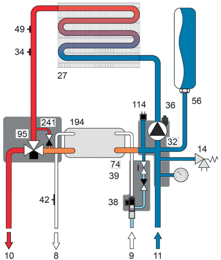
Рис. 15 Гидравлический контур
