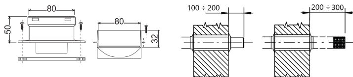
Труба подачи воздуха Труба дымоудаления
