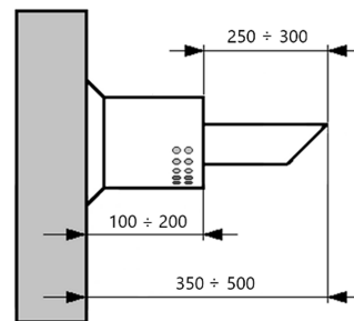
Рис.13а. "Вылет" трубы коаксиального дымохода
