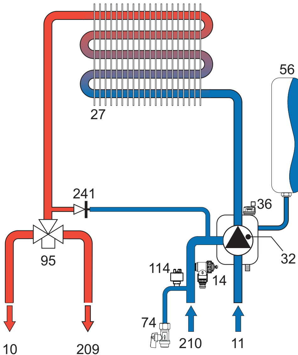
Рис. 45- Контур отопления
