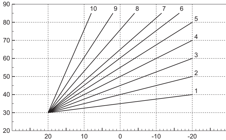
рис. 22- Компенсационные кривые
