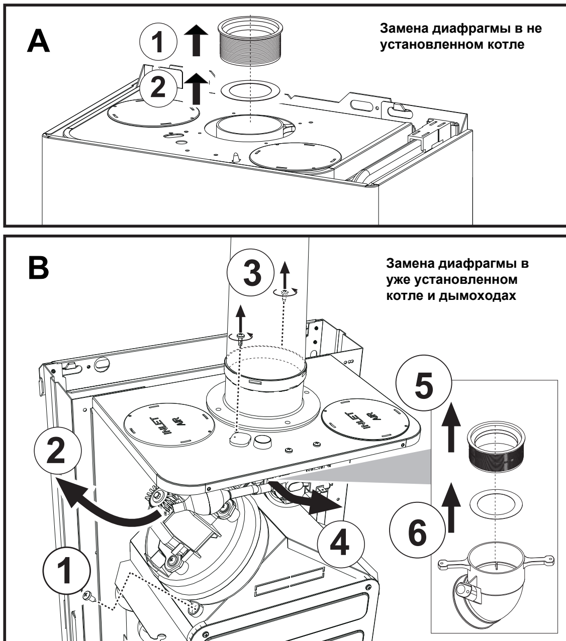
рис. 26- Замена диафрагмы
