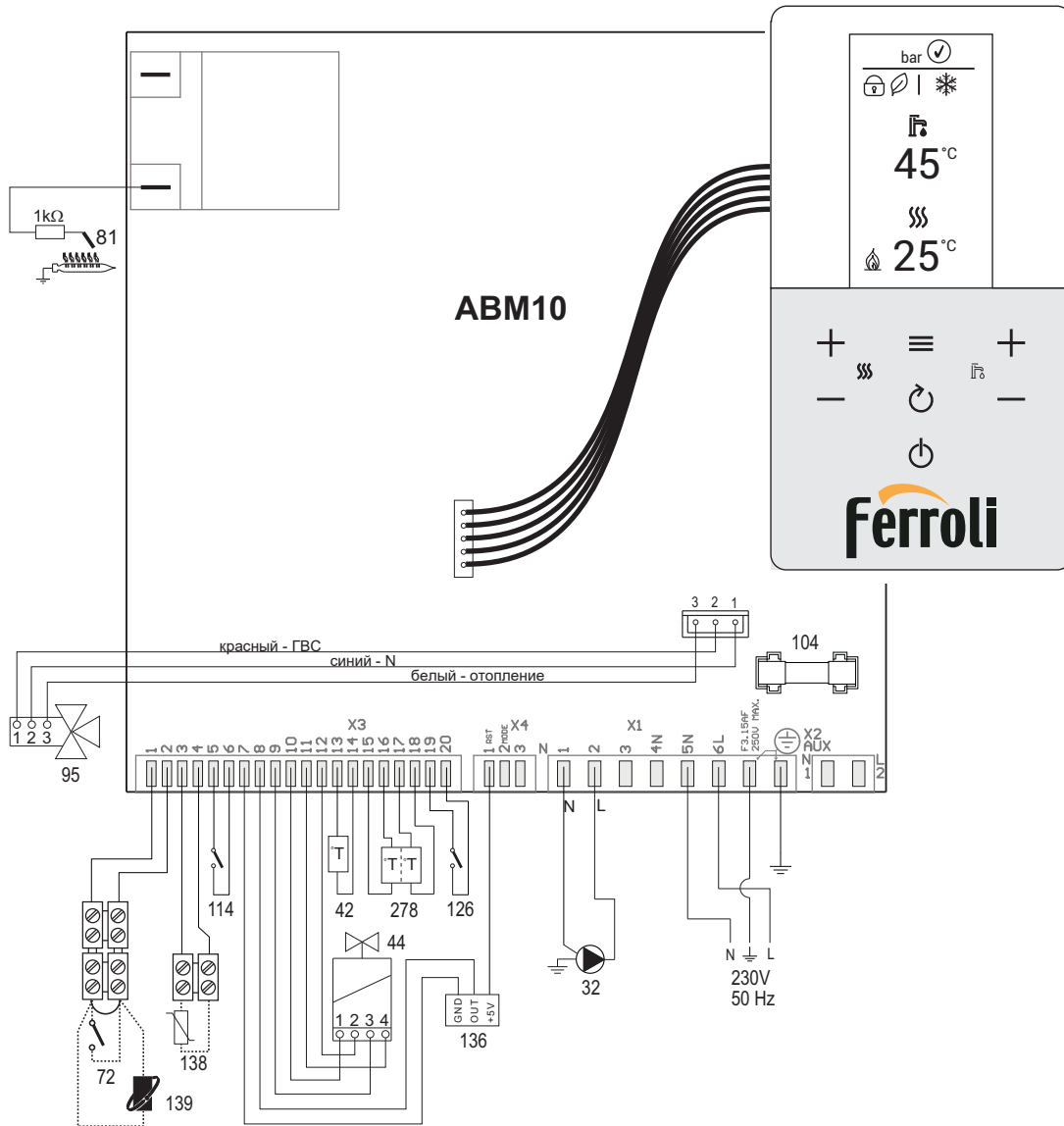
рис. 39- Электрическая схема
