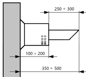
Рис. 21б. "Вылет" оголовка коаксиального дымохода
