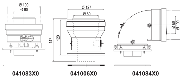
Рис. 21а. "Стартовые" аксессуары коаксиального дымохода
