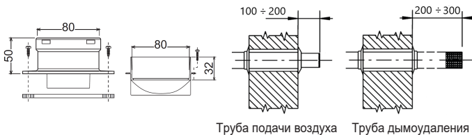
Рис. 11а. "Стартовые" элементы раздельного дымохода, арт 010011X0
