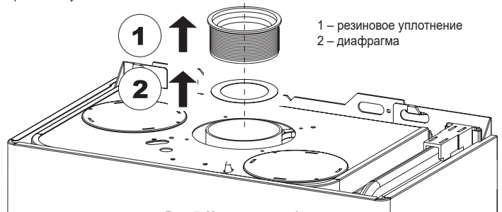
Рис. 7. Установка диафрагмы
