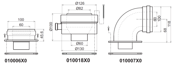
Рис. 9а. "Стартовые" элементы коаксиального дымохода
