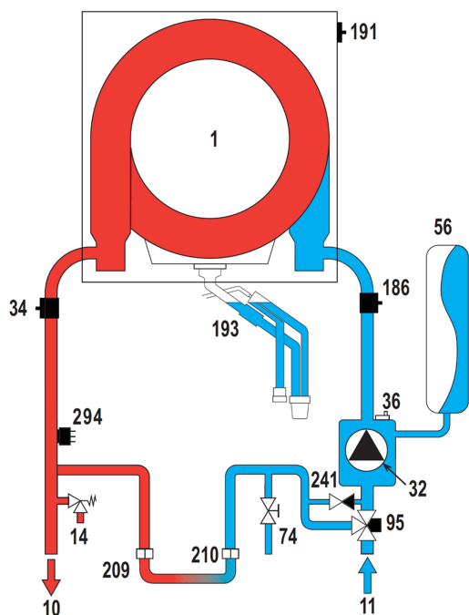
рис. 76- Гидравлический контур
