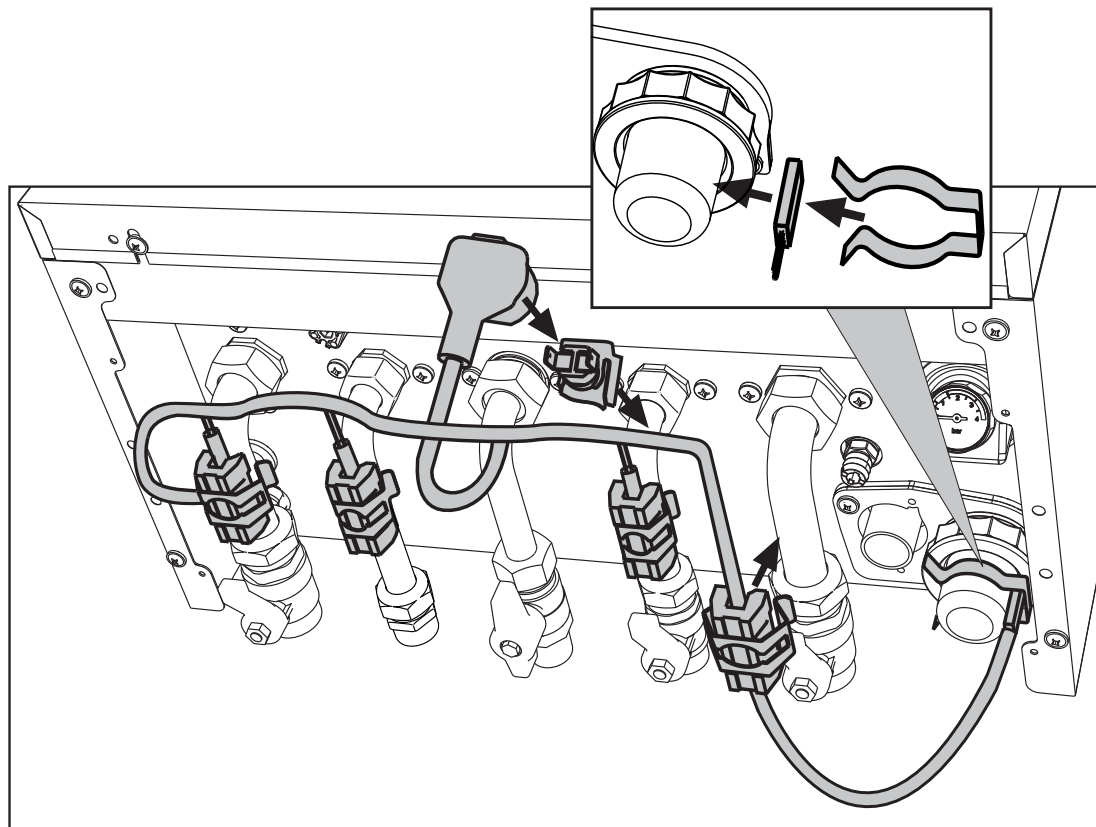
рис. 49- Противообледенительный комплект
