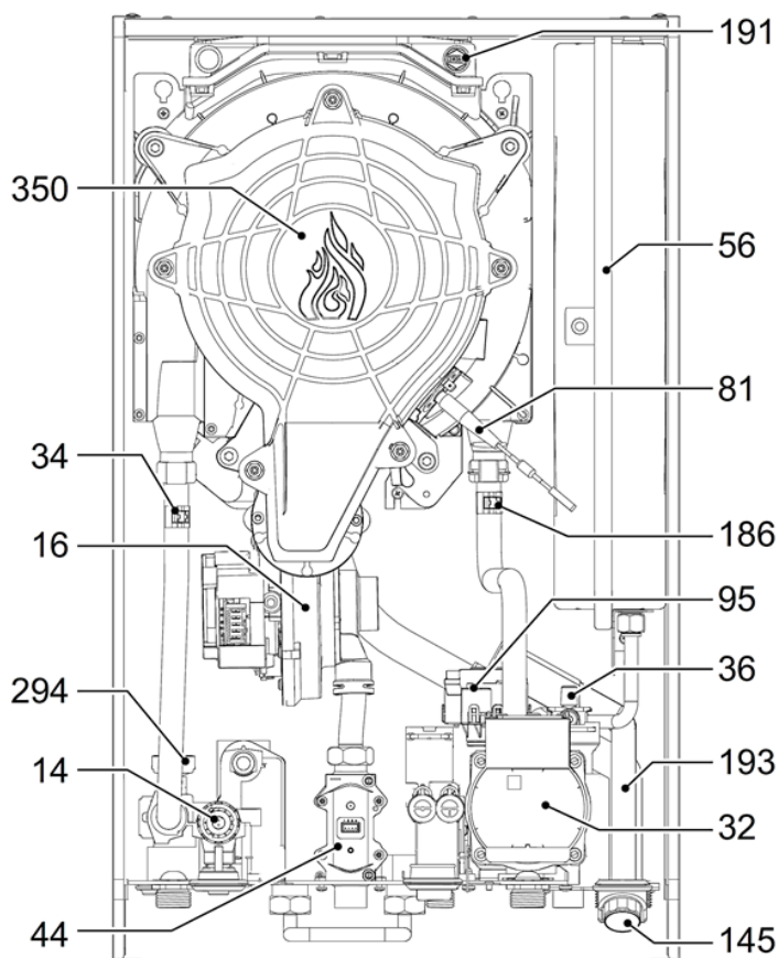
рис. 75- Общий вид
