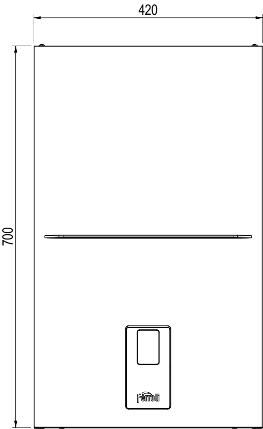
рис. 71- Вид спереди
