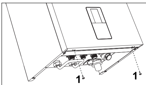
рис. 56- Открытие передней панели
