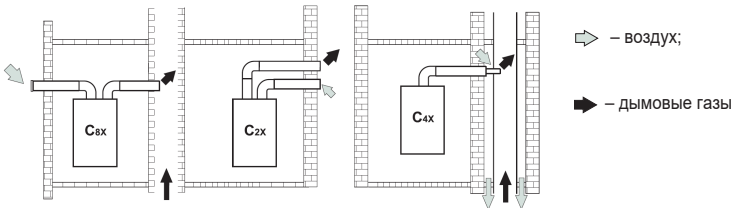
Рис. 12. Примеры подсоединения к дымоходам
