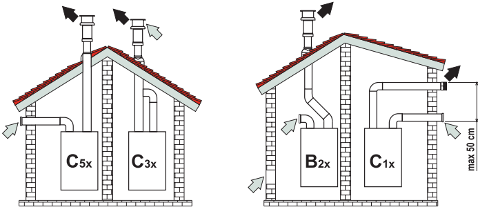
Рис 10. Примеры присоединения с помощью раздельных труб
