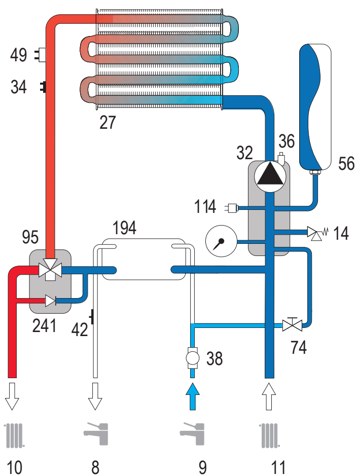
Рис. 18. Контур отопления
