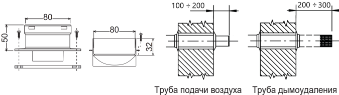
Рис. 11а. "Стартовые" элементы раздельного дымохода, арт 010011X0
