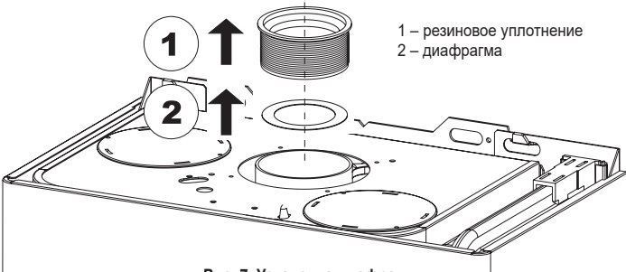
Рис. 7. Установка диафрагмы
