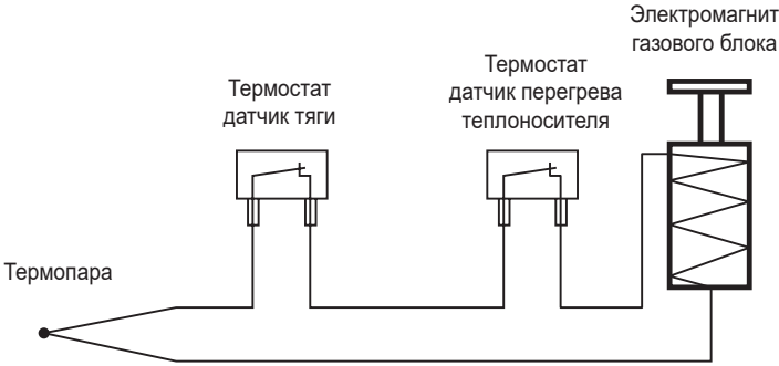
Рис. 4. Электрическая схема соединения в цепи термопары
