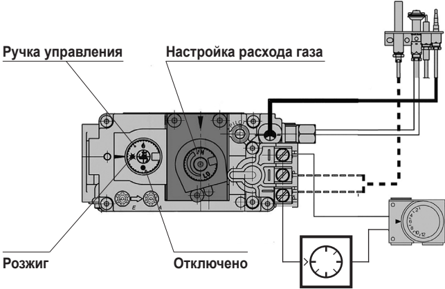
Рис. 11. Схема подключения комнатного термостата
