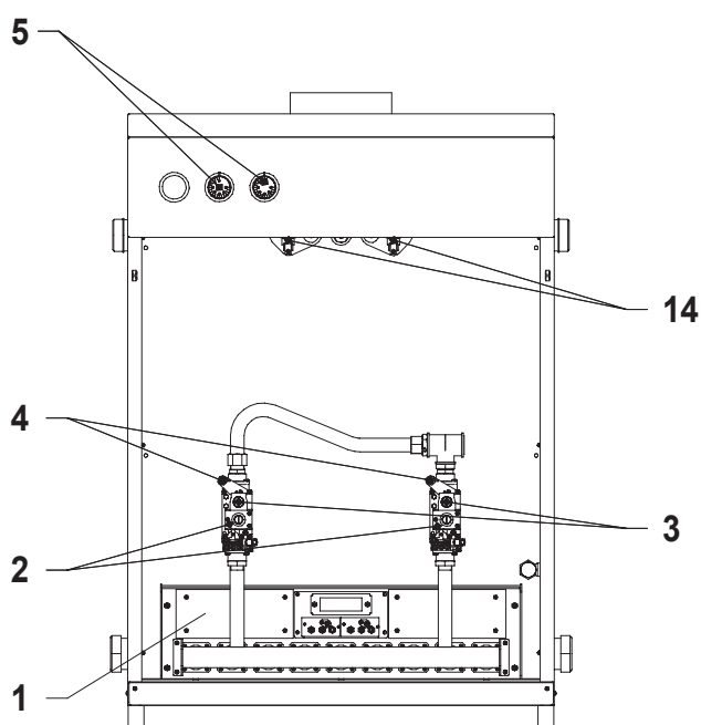
Рис. 3. Особенности котла TORINO 100 с двумя газовыми блоками 820 NOVA mV
