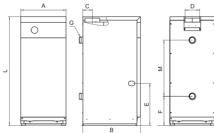
Рис. 1. Общий вид, габаритные и присоединительные размеры котлов
