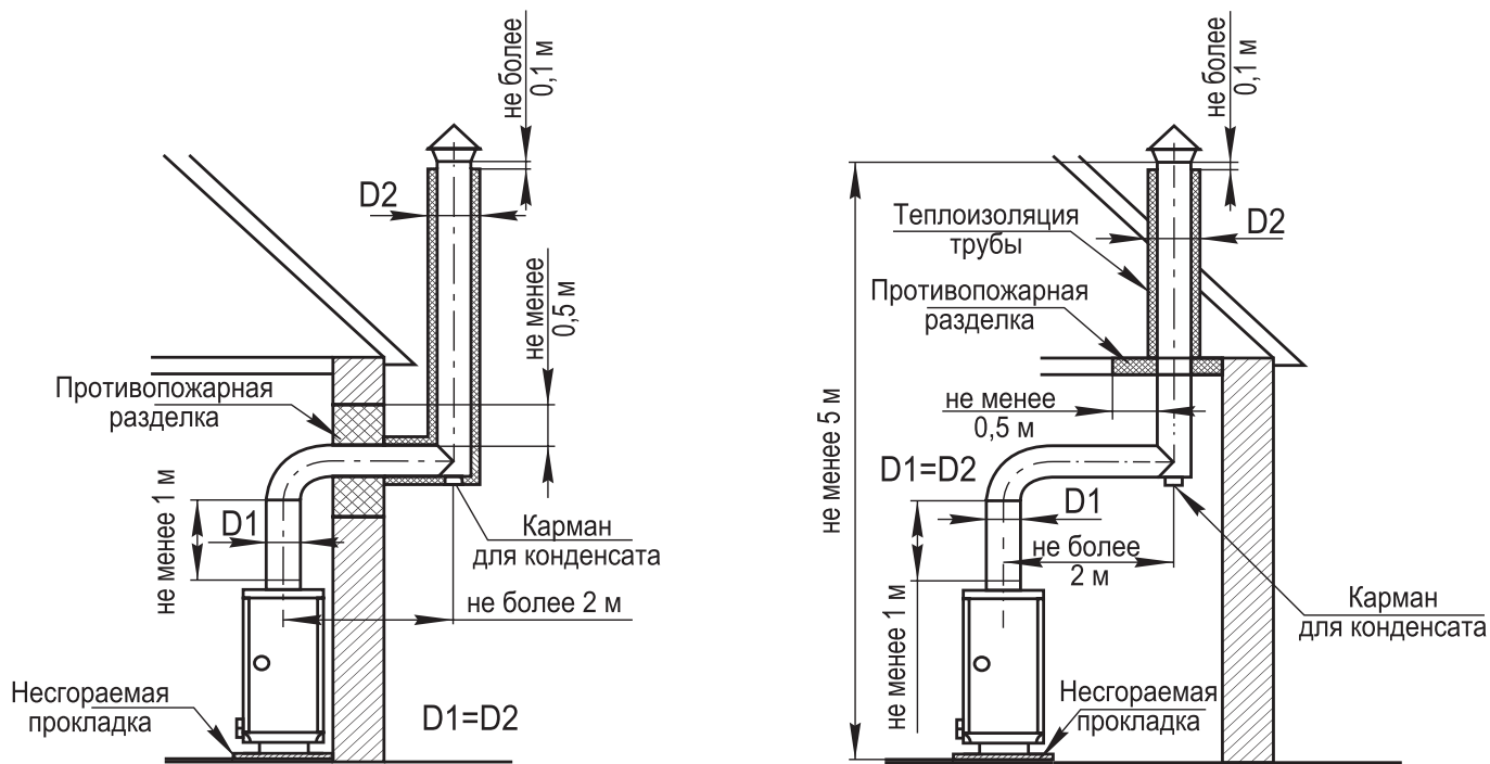
Рис. 7. Схема установки дымовой трубы с выводом через стену и с выводом через потолочное перекрытие
