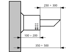
Рис. 8а. "Стартовые" элементы коаксиального дымохода
