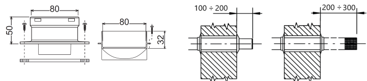
Рис. 9а. "Стартовые" элементы раздельного дымохода, арт 010011Х0
