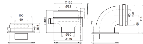
Рис. 8а. "Стартовые" элементы коаксиального дымохода
