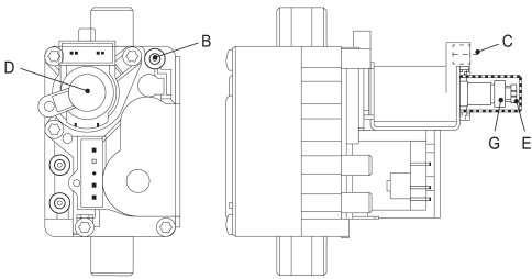
Рис. 13. Газовый клапан
