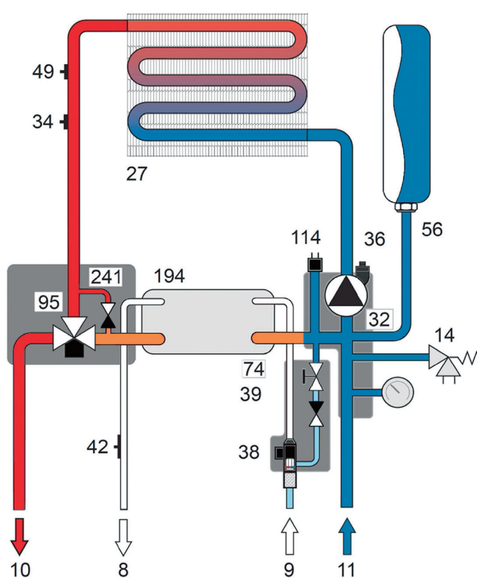
Рис. 14 Гидравлический контур
