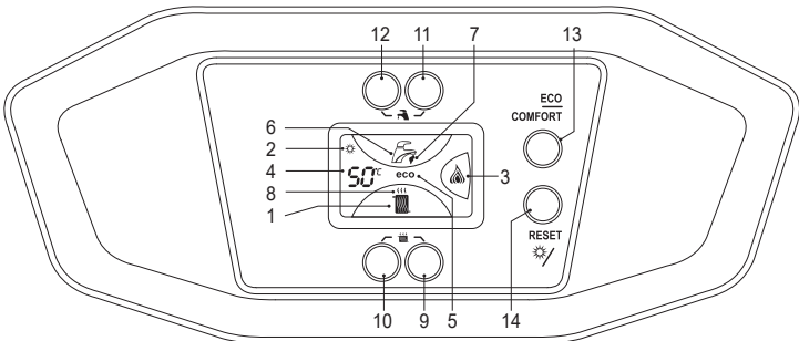
Рис.1. Панель управления
