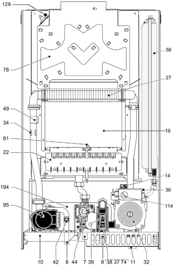
Рис. 18а. Конструкция VITABEL C24
