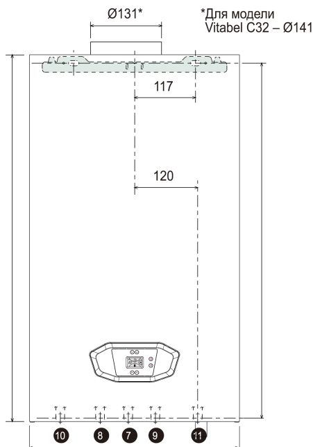
Рис. 17. Установочные размеры моделей "С"
