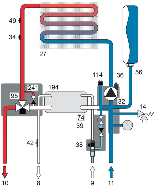
Рис. 19а. Отопительный контур
