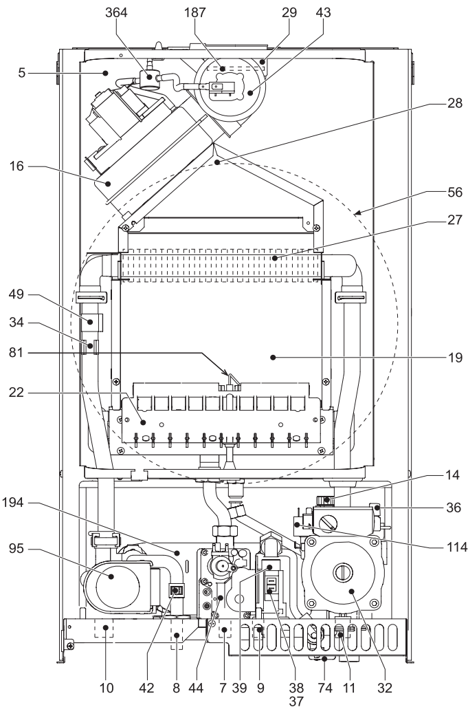
Рис. 18b. Конструкция VITABEL F32-40
