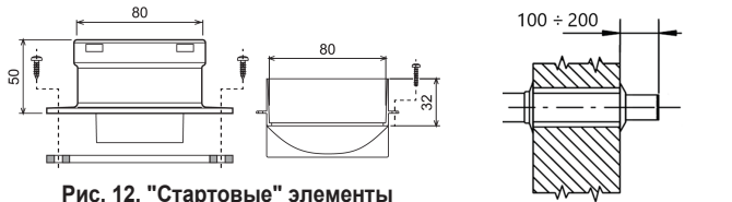
Рис. 12. "Стартовые" элементы раздельного дымохода, арт 010011X0
