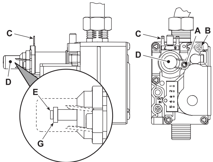
Рис. 15. Газовый клапан
