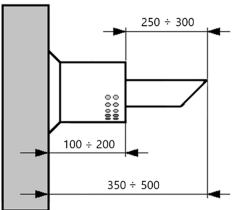
Рис. 9а. "Стартовые" элементы коаксиального дымохода
