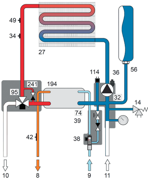
Рис. 19b. Контур ГВС
