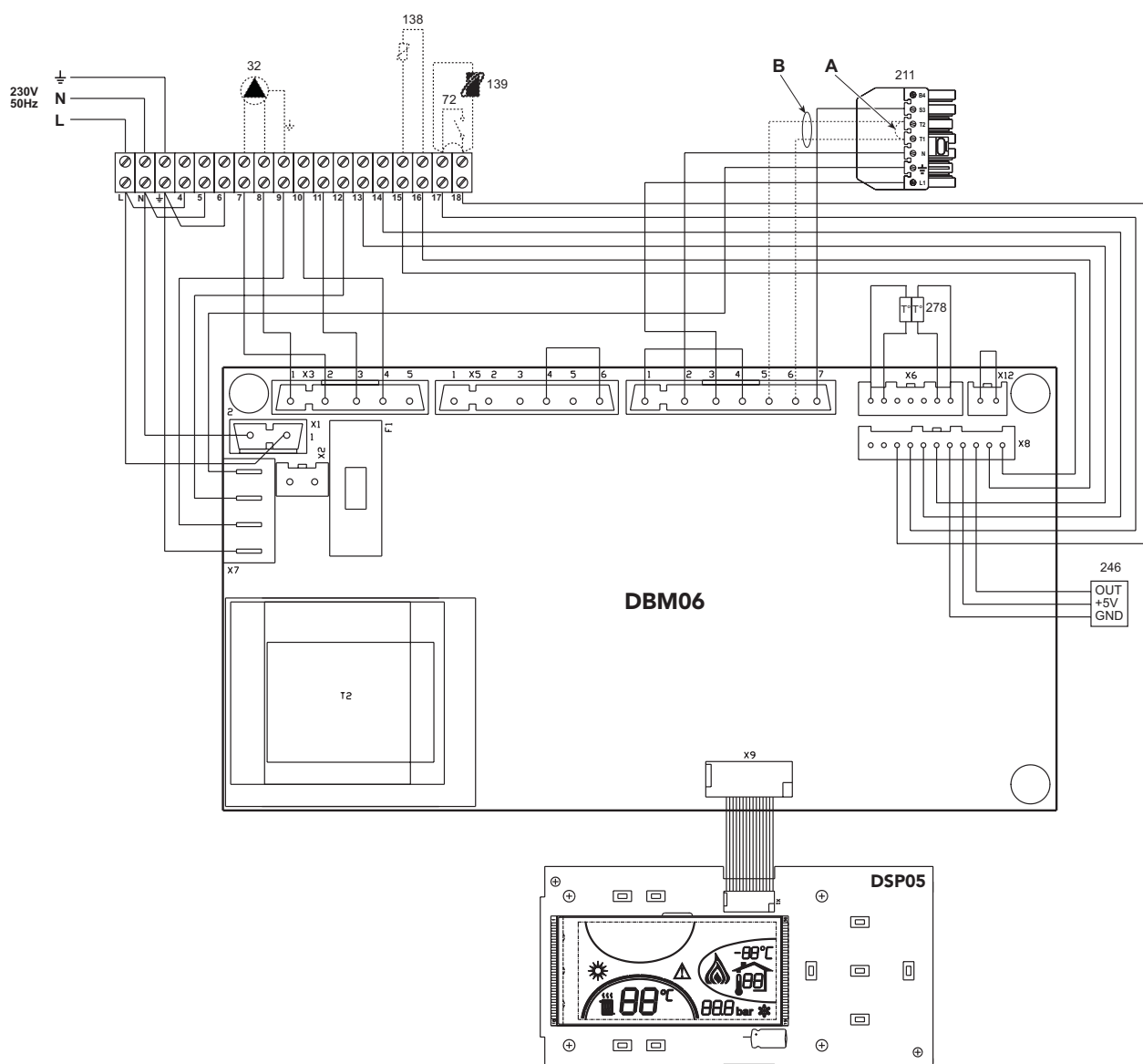
рис. 18 - Электрическая схема
