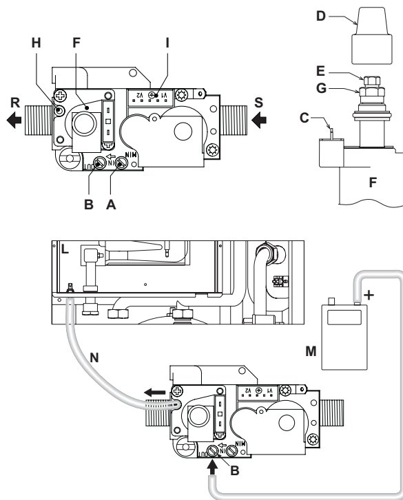
рис. 27 - Газовый клапан
