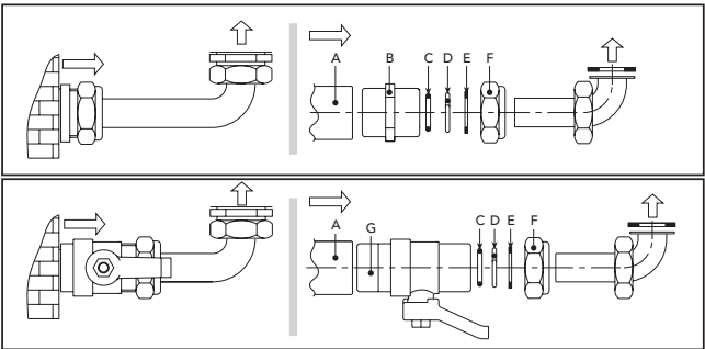
рис. 18 - Соединительный комплект
