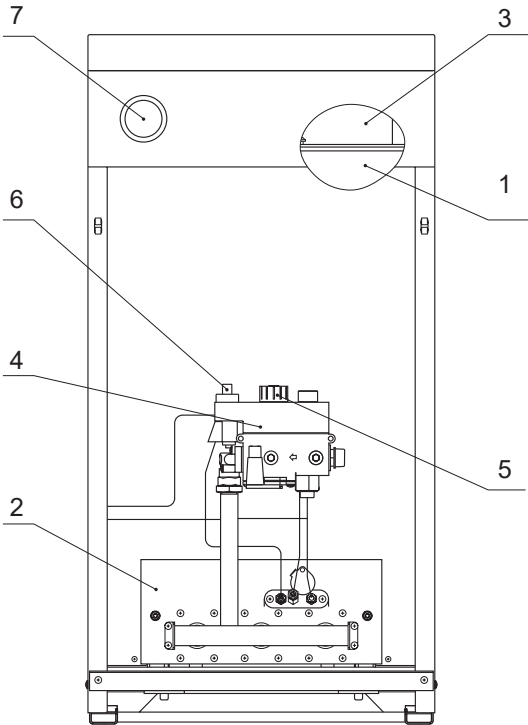
Рис. 3. Особенности котла с газовым блоком 710 MINISIT Модели котлов TORINO CLASSIC 25; 30
