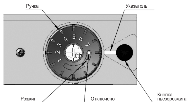
Рис. 9. Элементы управления на газовом блоке управления 630 EUROSIT
