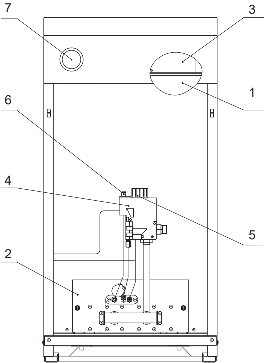
Рис. 2. Особенности котла с газовым блоком 630 EUROSIT Модели котлов TORINO CLASSIC 10; 12,5; 16; 20
