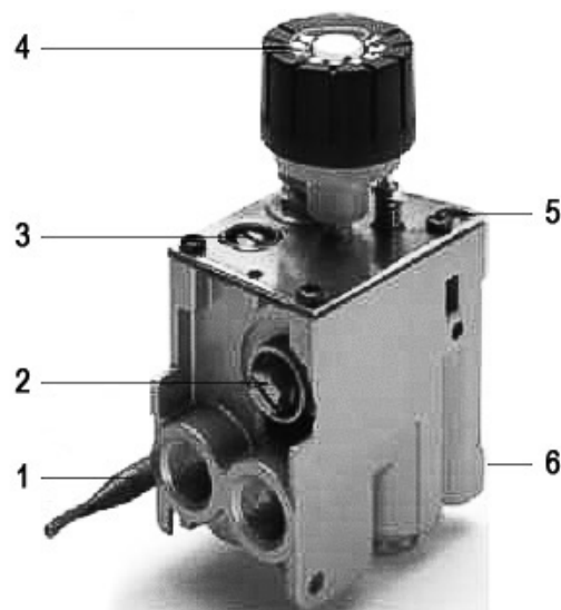
Рис. 11. Газовый блок 630 EUROSIT
