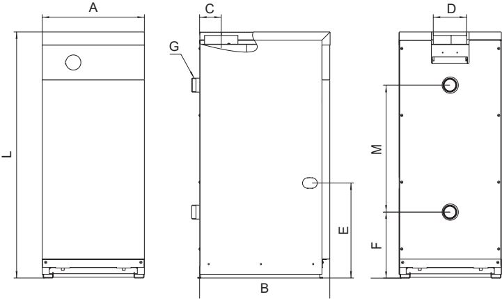
Рис. 1. Общий вид, габаритные и присоединительные размеры котлов
