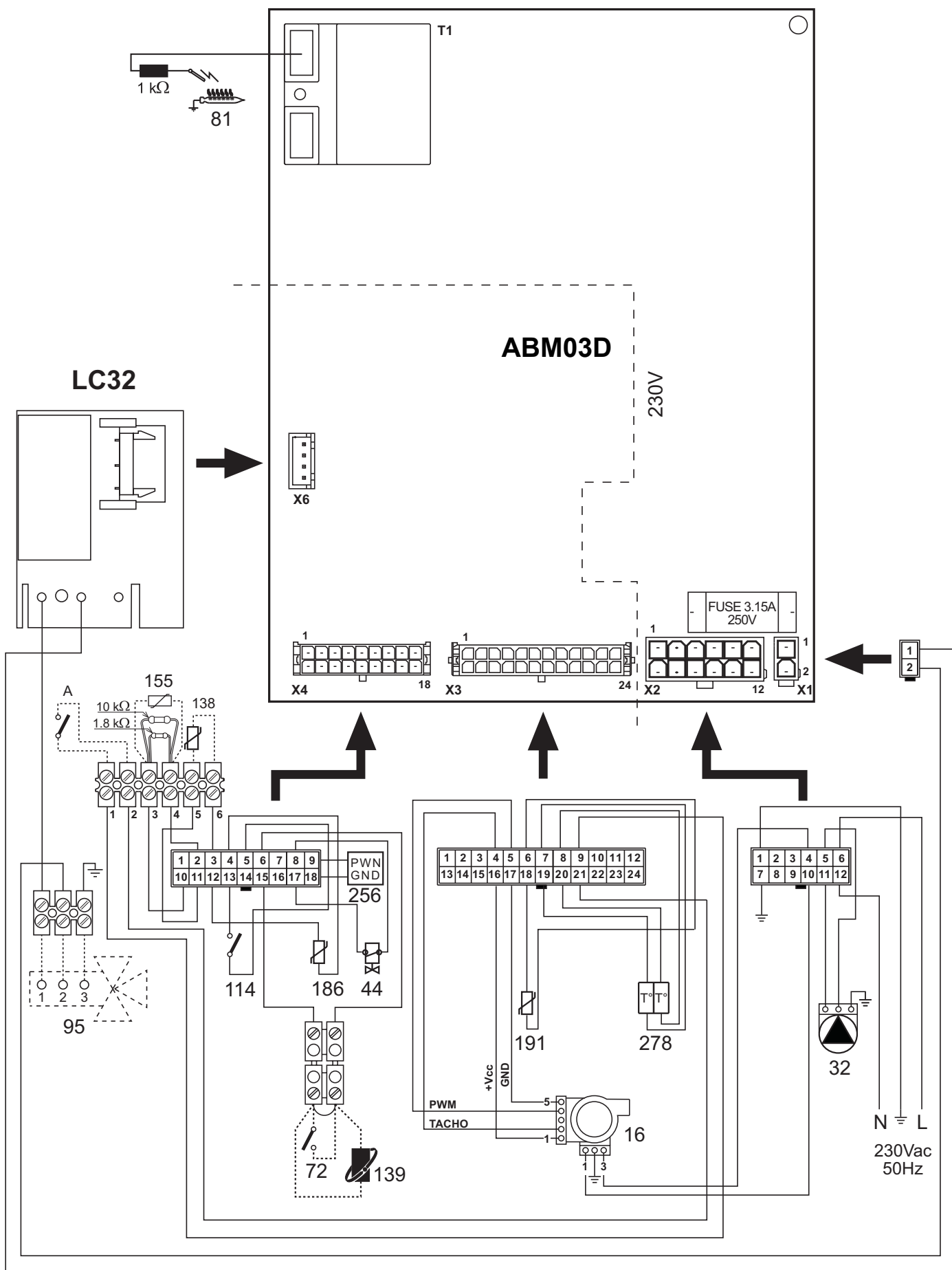
fig. 29 - Schemă electrică
