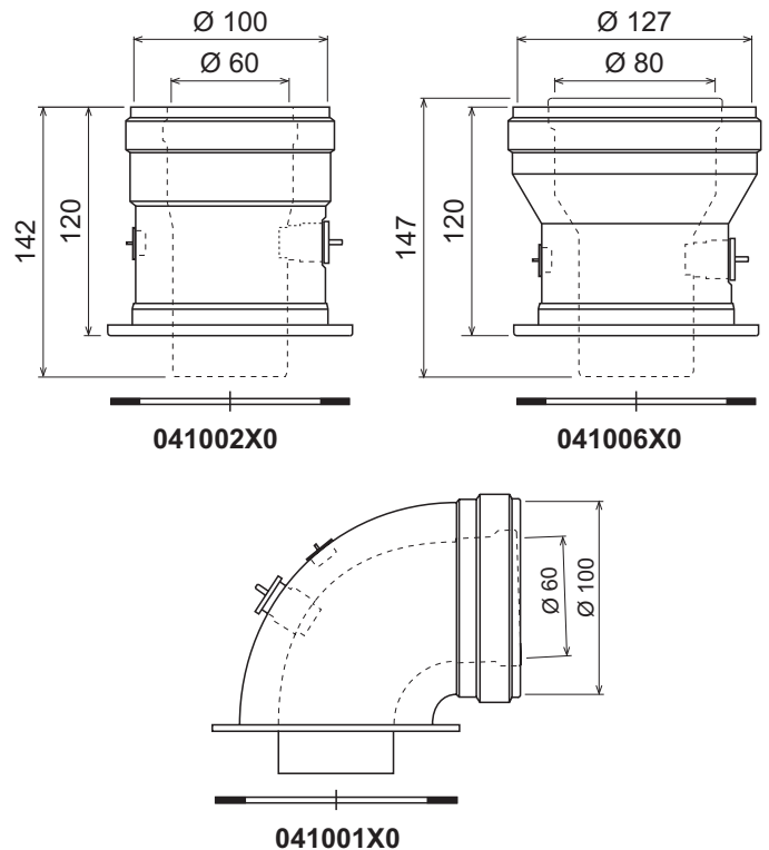
fig. 16 - Accessori di partenza per condotti coassiali
