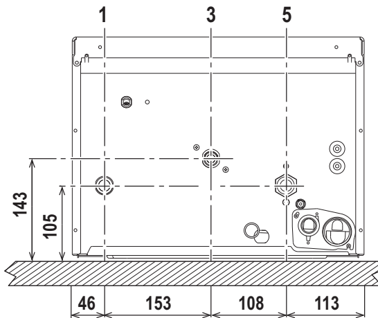
рис. 12 - Гидравлические соединения
