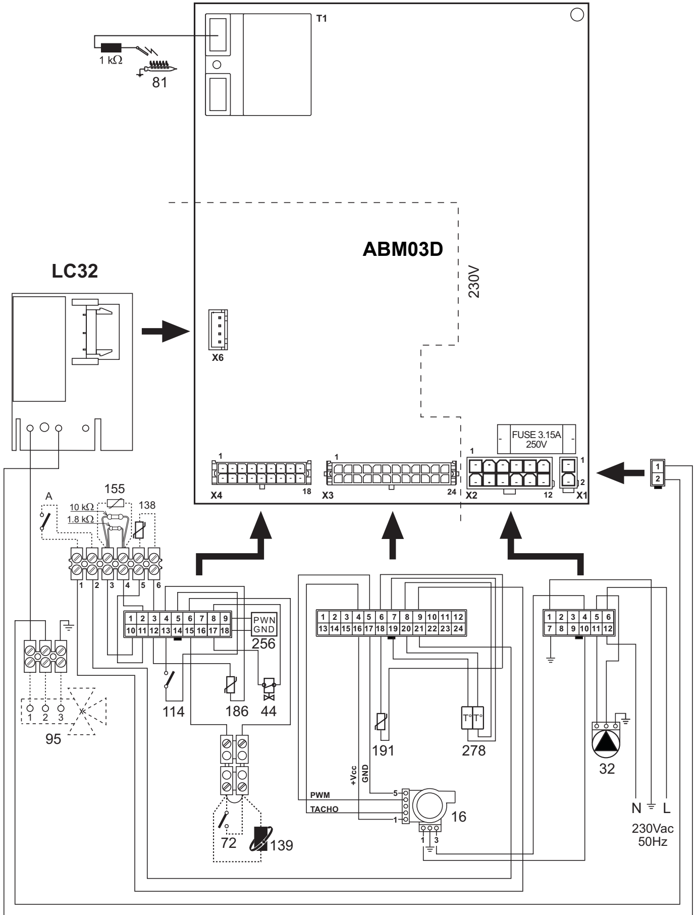
fig. 29 - Schéma électrique
